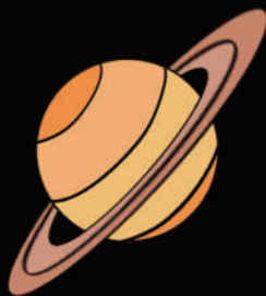
Saturnus
